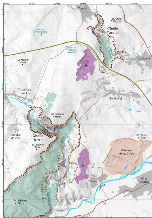
Fig. 2. Forme exocarstice
